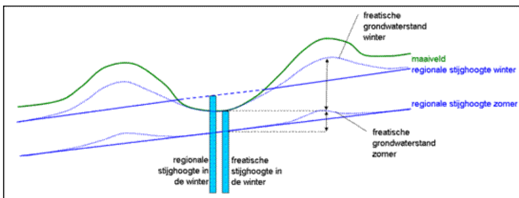
Figuur 3.8 Schematische voorstelling regionale en lokale kwel, situatie Charaven (deelgebied Stelkampsveld).
