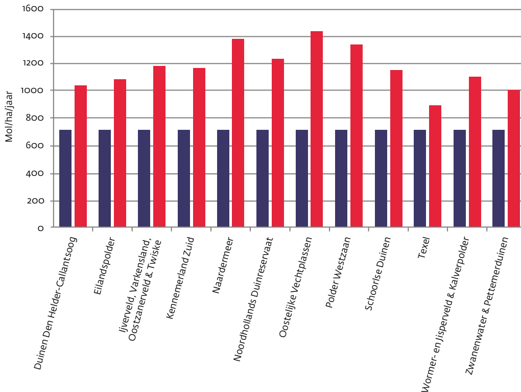
Figuur 3: gemiddelde stikstofdepositie in de Noord-Hollandse Natura 2000-gebieden (rood) en de KWV van de meest kritische habitat in deze gebieden (blauw).
