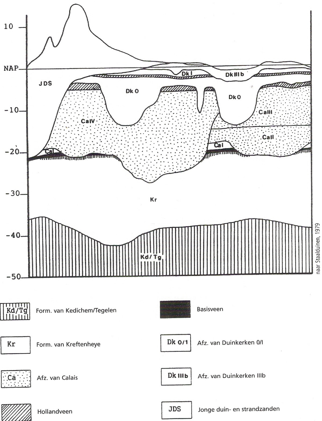
Figuur 3-7. Geologisch profiel (van Steenis, 2006, naar Staaldunin, 1979).
