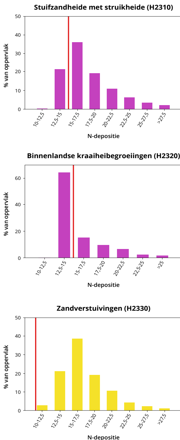
Figuur 4.7. Verdeling van de stikstofdepositie per 2,5 kg N/ha/jaar-klasse voor stuifzandheide met struikheide (H2310), binnenlandse kraaiheidebegroeiingen (H2320) en zandverstuivingen (H2330) als percentage van het totaal oppervlak. De rode lijn geeft de KDW van het type weer.
