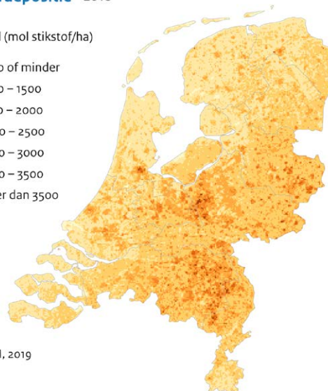
Figuur 3.5. Verdeling van de stikstofdepositie over Nederland in 2018.
